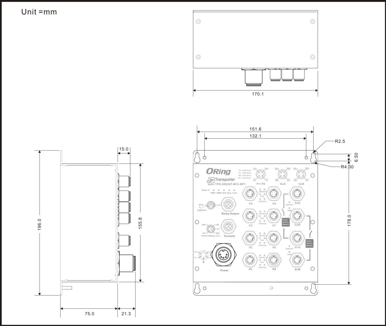
TPS-3082GT-M12-BP1 / TPS-3082GT-M12-BP1-24V Dimension
