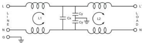
电气原理图(Electrical Schematic) : 37
