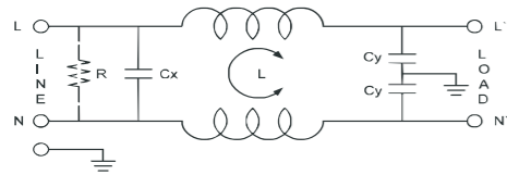
电气原理图(Electrical Schematic) : 37
