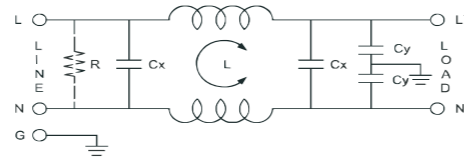
电气原理图(Electrical Schematic) : 38
