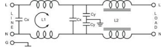
电气原理图(Electrical Schematic) : 38
