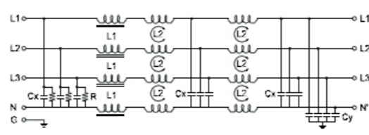
电气原理图(Electrical Schematic) : 94
