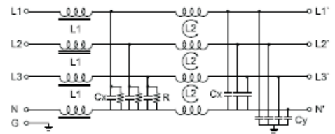
电气原理图(Electrical Schematic) : 93
