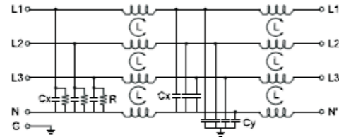
电气原理图(Electrical Schematic) : 94
