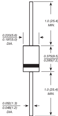
DO-201AD
