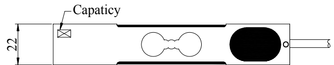
主視 (Front View)
