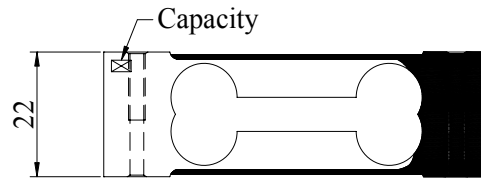
主视(Front View)
