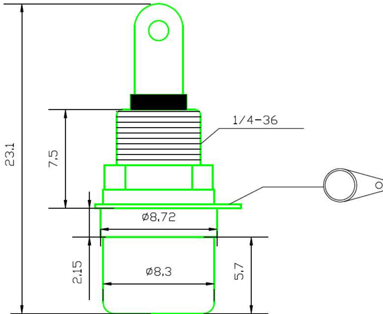
CONNTERM RCA-XP-AM-CT
