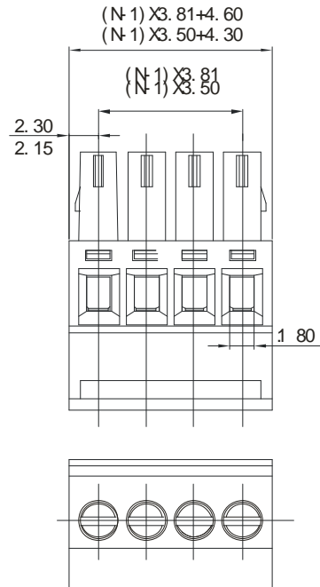
15EDGKA-3.5 15EDGKA-3.81
