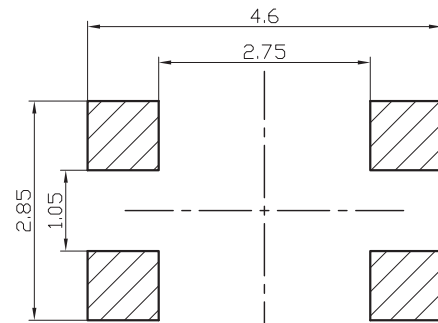
安装参考图 P.C.B layout
