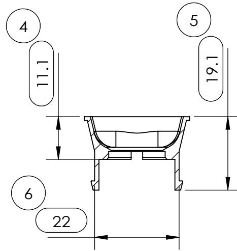
剖面图 A-A
